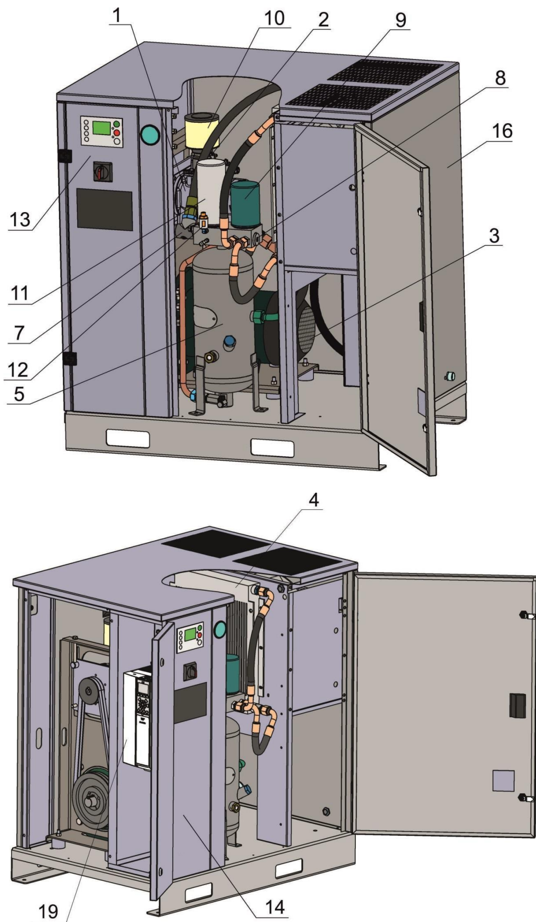
Рисунок 1.6 – Общий вид компрессорной установки ВК20Т-15
