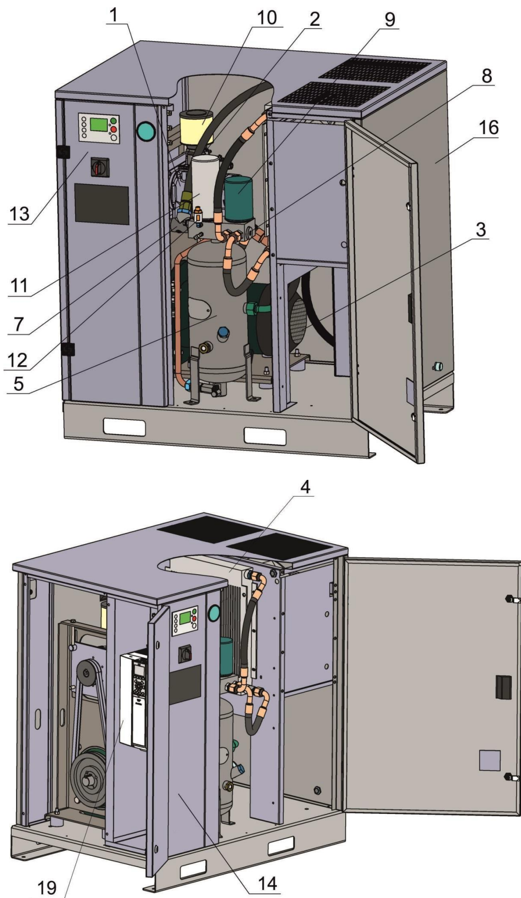
Рисунок 1.6 – Общий вид компрессорной установки BK20T-15
