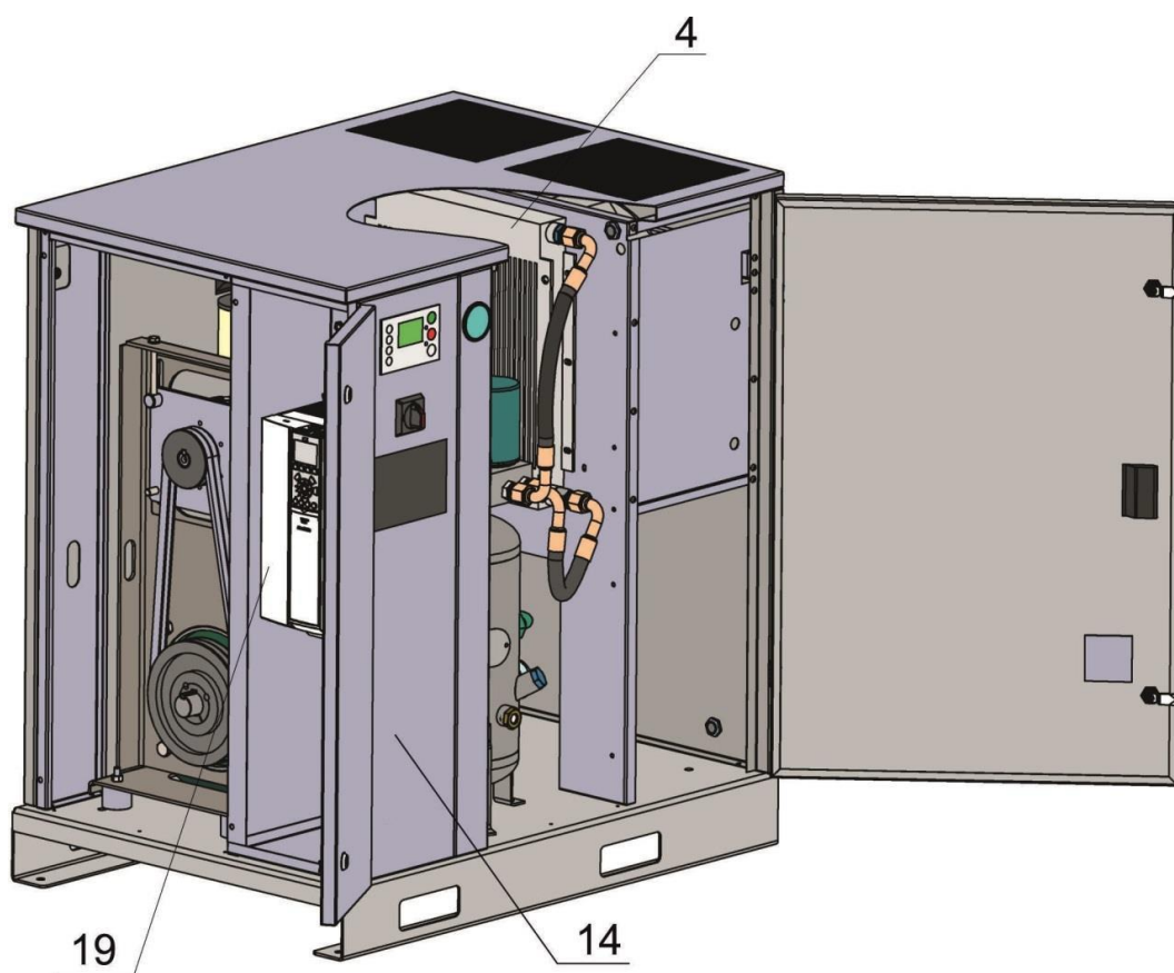
Рисунок 1.6 – Общий вид компрессорной установки BK20T-15
