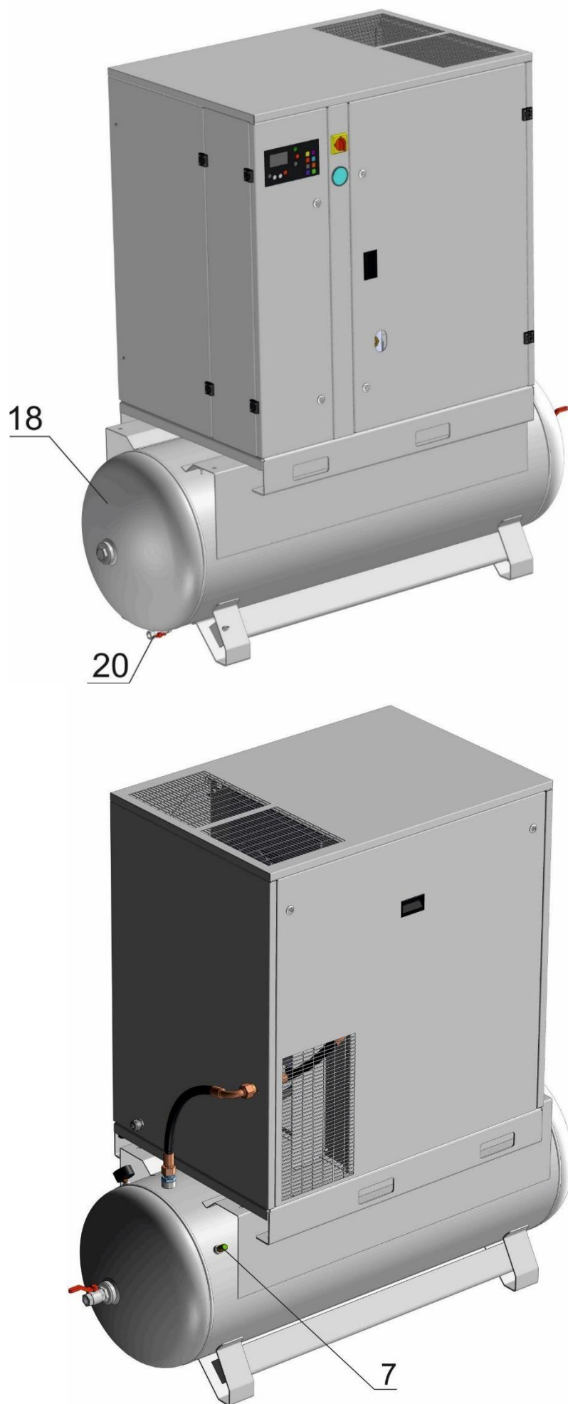
Рисунок 2 – Общий вид компрессорных установок BK25T-...-500(BC), 30T-...-500(BC)
