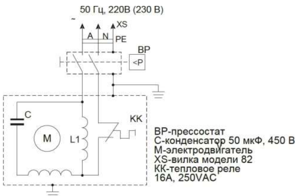
Рисунок А.1 - Схема электрическая принципиальная компрессора СБ4-F22А
